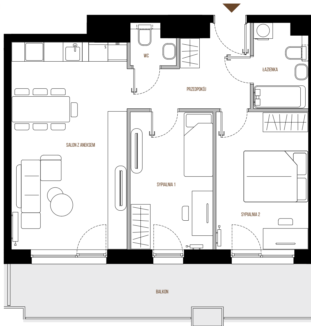
RZUT LOKALU
