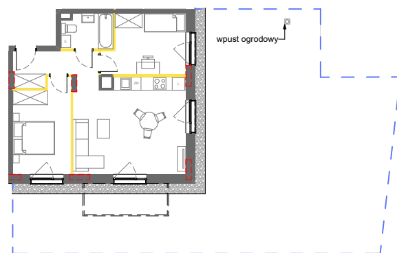
SCHEMAT MIESZKANIA
