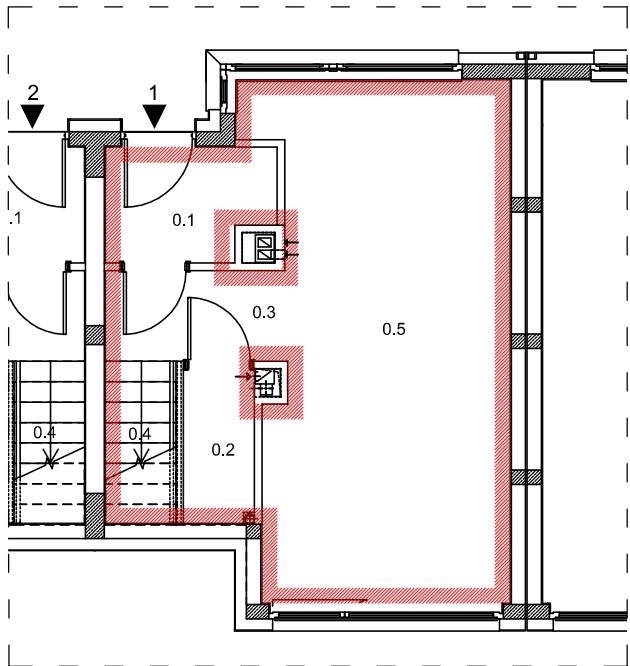
RZUT PARTERU BUDYNKU NR 9A LOKAL MIESZKALNY NR 1
