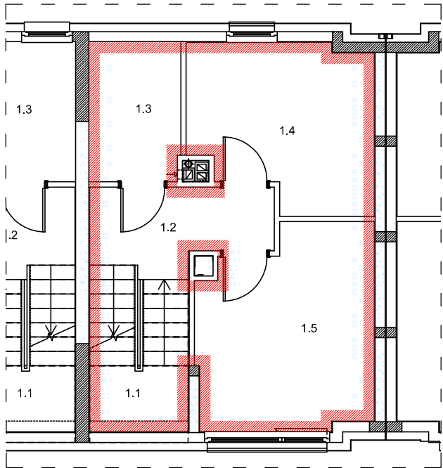
RZUT PIĘTRA I-GO BUDYNKU NR 9A LOKAL MIESZKALNY NR 1
