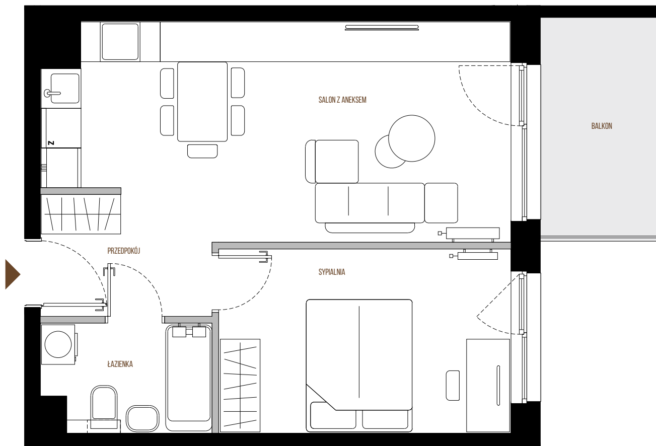
RZUT LOKALU
