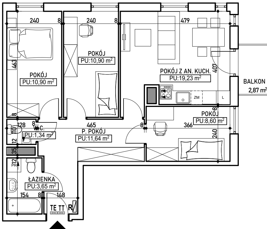
RZUT KONDYGNACJI 2 PIĘTRA BUD. B Z ZAZNACZENIEM LOKALU MIESZKALNEGO
