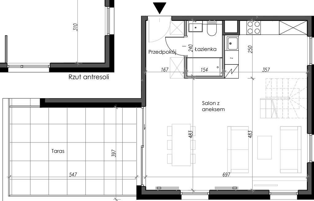
Rzut 4 piętra
