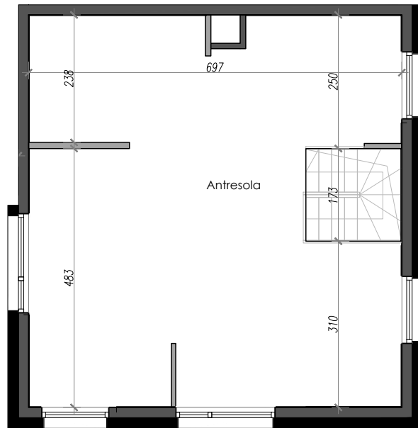
Rzut antresoli
