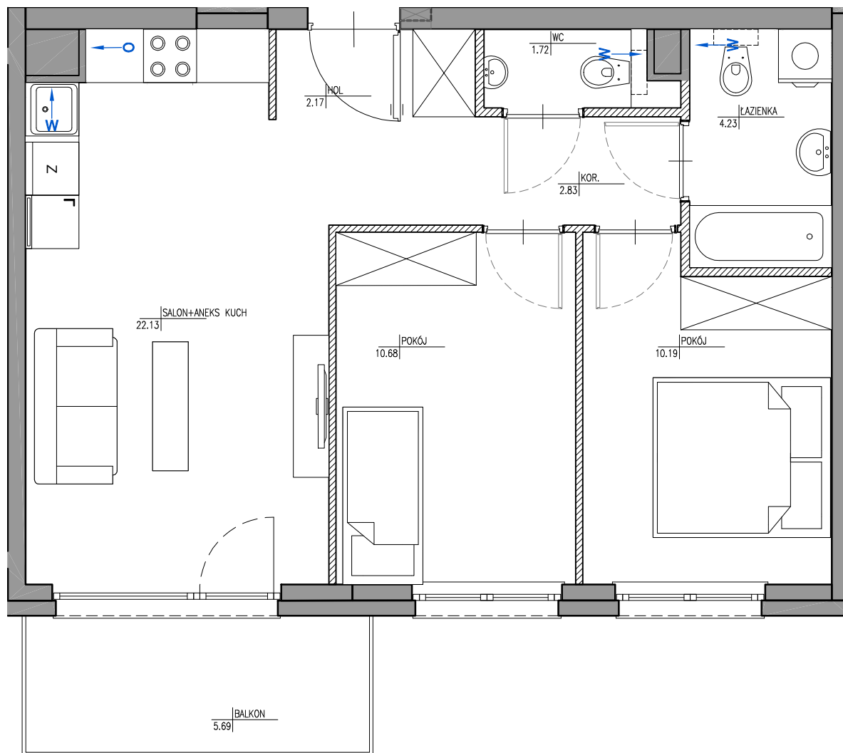
SCHEMAT LOKALU NA RZUCIE
