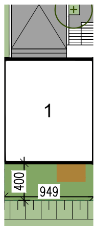
WYMIARY OGRÓDKA
