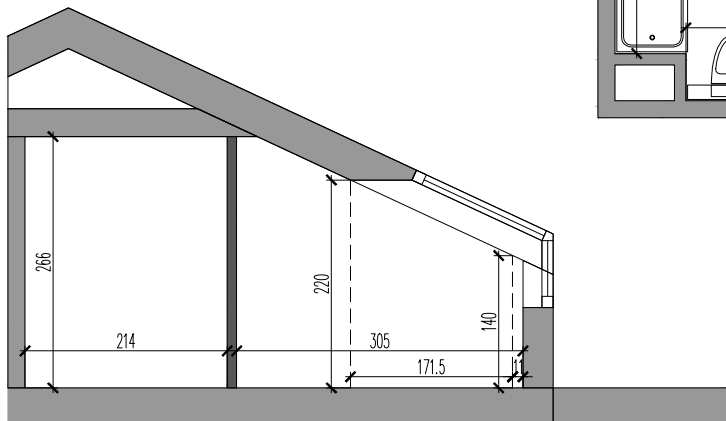
PRZEKRÓJ A-A
