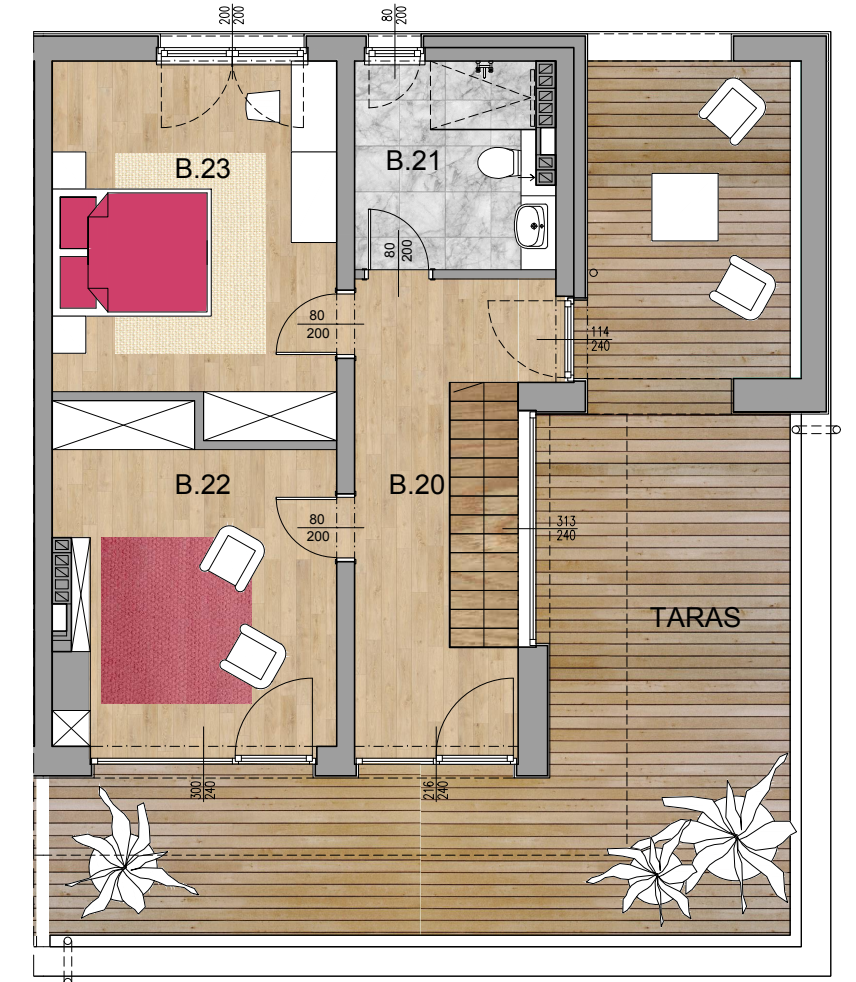
RZUT 2 PIETRA
